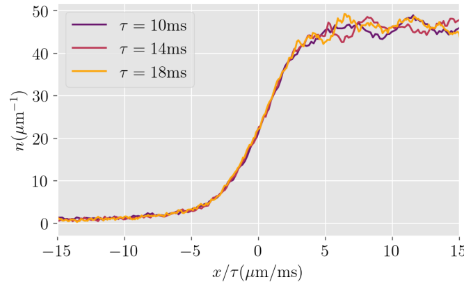
FIGURE 6.1 – Profils de densité mesurés pour différents temps t , représentés en fonction de la variable x/\tau . L'excellent recouvrement des courbes confirme l'auto-similarité et la dynamique balistique.
